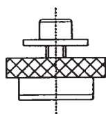
10368 eindstop met rubber arrêt avec caoutchouc endcap with rubber
