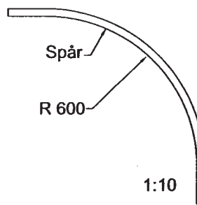
10365 Bocht KM (enkel in combinatie met EPM profiel 10347) Courbe KM (ne peut s'utiliser qu'avec le profilé EPM 10347) Bend KM (only in combination with EPM profile 10347)
