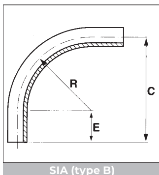
SIA (type B)
