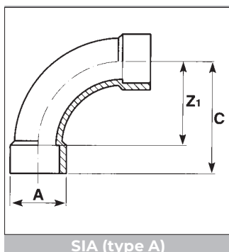
SIA (type A)
