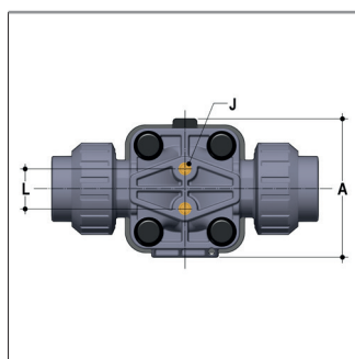
VMOC - DN 80-100
