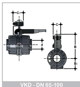
VKD - DN 65-100
