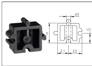
TYPE D
