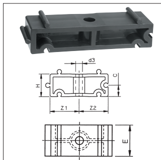
TYPE E
