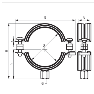
BIFIX 5000 G2
