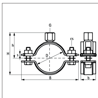
BIS HD1501
